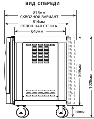
ВИД СБОКУ: ДВОЙНАЯ ГНУТАЯ ДВЕРЬ, СПЛОШНАЯ ЗАДНЯЯ СТЕНКА
